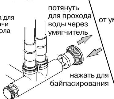
Байпасный вентиль
